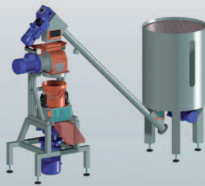
Pellettizzatrice + Raffinatore + Mini Silo di Carico
