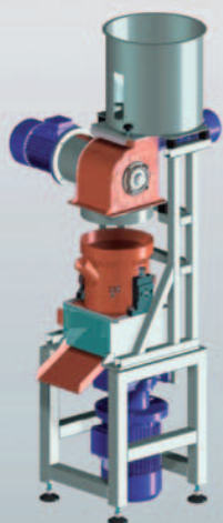
Pellettizzatrice + Raffinatore + Dosatore
